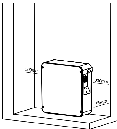
Installazione a pavimento
