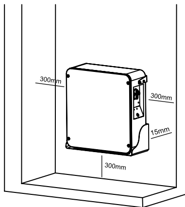
Installazione a parete
